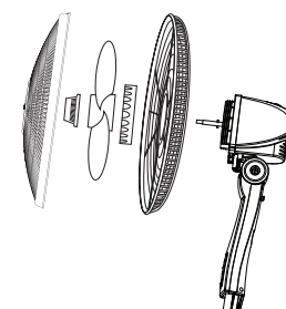
1. Ensamble la cabeza del ventilador
